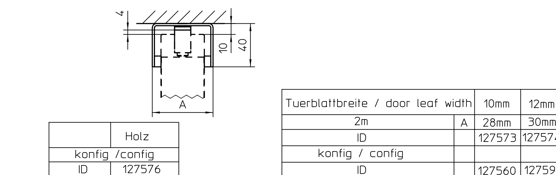
Abdeckkappe Wandbefestigung Deckenfuehrung Gealan Cover cap wall mounting Gealan
