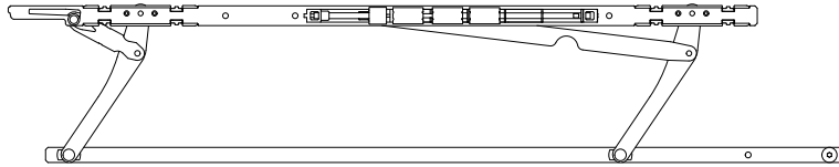
26 Gleitschere
