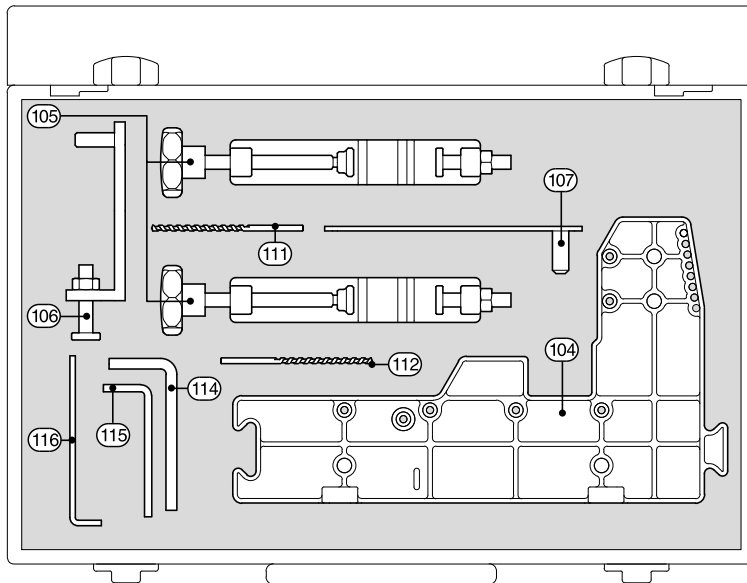
Lehrenkoffer
