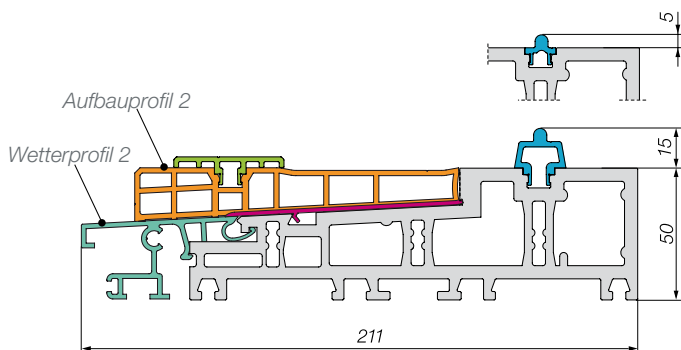
Mit Aufbauprofil 2 und Wetterprofil 2 für Flügelstärken ab 80 mm. Wahlweise auch mit flacher Laufschiene für barrierefreies Wohnen.
