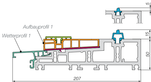
Mit Aufbauprofil 1 und Wetterprofil 1 für Flügelstärken bis 79 mm. Wahlweise auch mit flacher Laufschiene für barrierefreies Wohnen.
